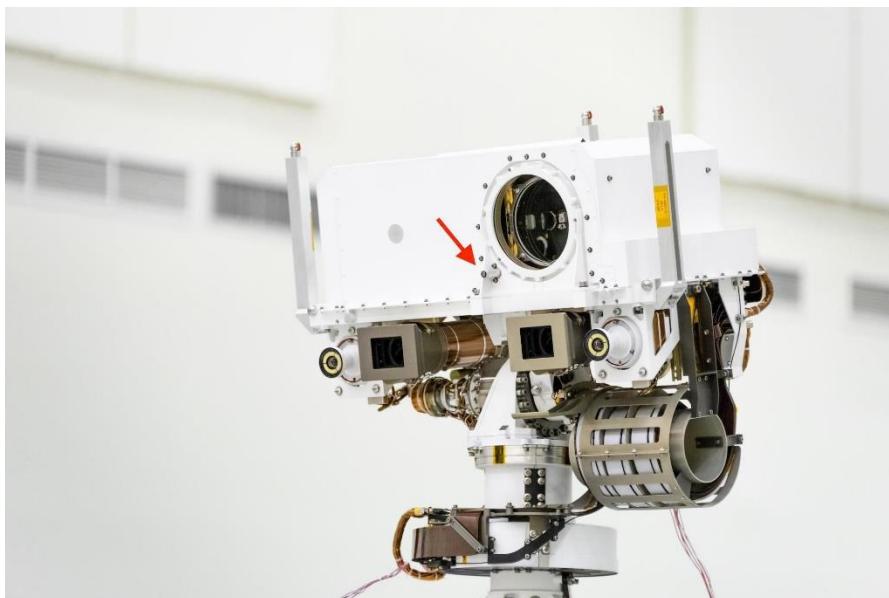
Le dispositif SuperCam du rover Perseverance. La flèche rouge pointe le microphone. Il ne mesure que 3,4 cm de long pour un poids plume de 13 grammes. © Nasa, JPL-Caltech
